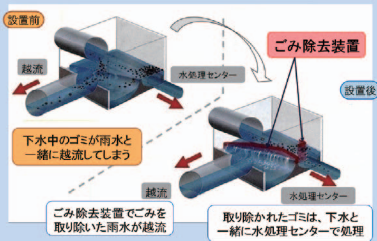
合流式下水道の改善 (ゴミ除去装置の設置)
